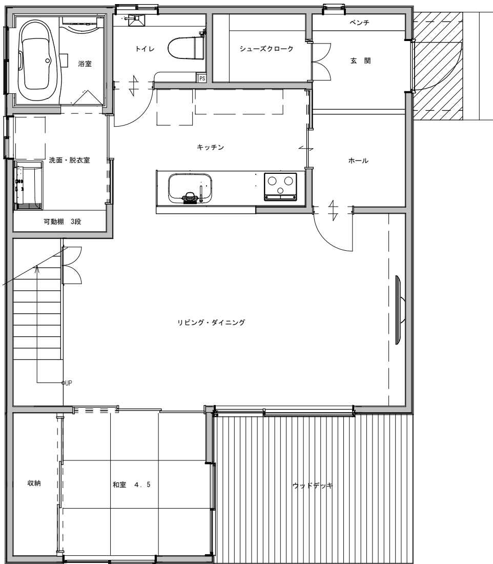
1階 平面図
