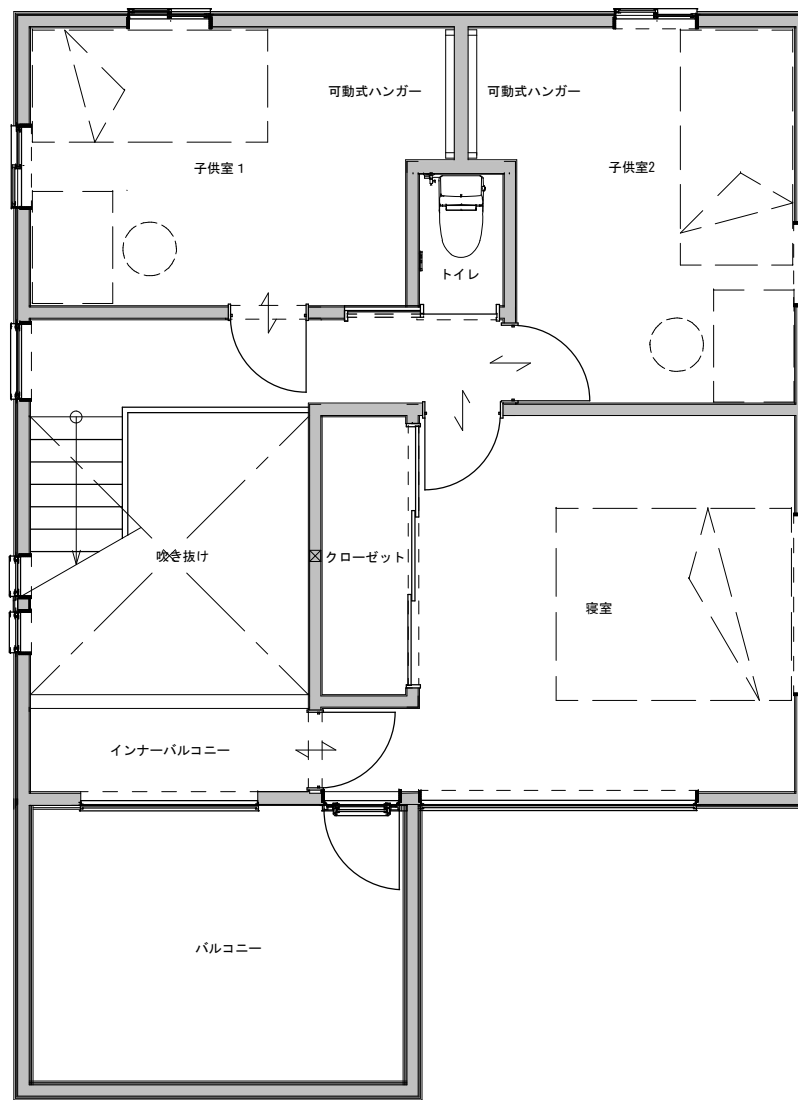
2階 平面図
